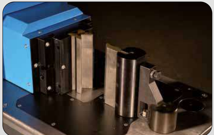
Outil de pliage
